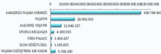
Erişim Grafiği
