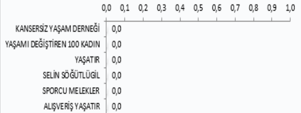
Süre Grafiği
